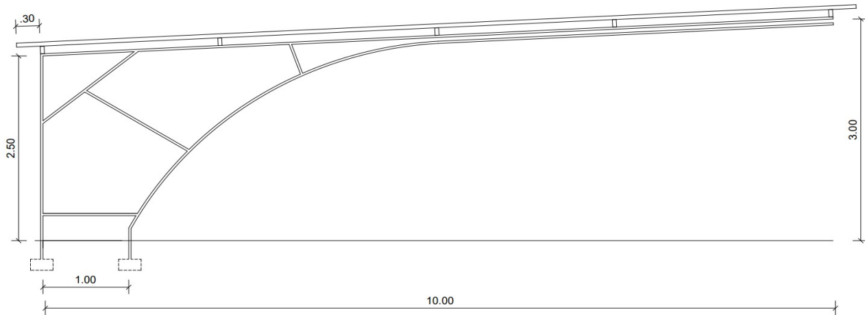
Figura 2: Elevação
